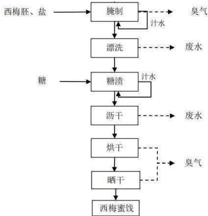
图2-2 西梅蜜饯生产工艺流程及产污环节图
