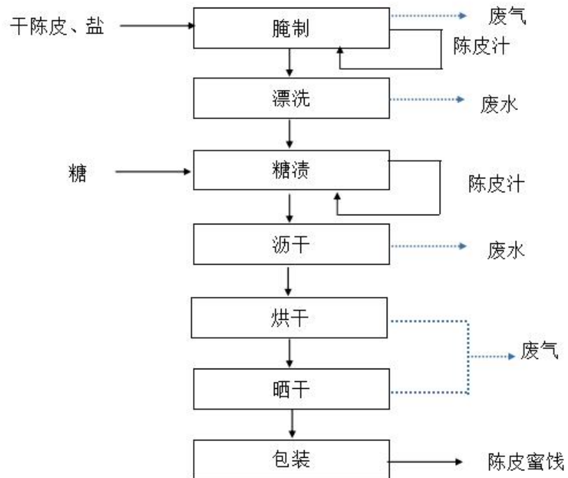
图2-3 陈皮生产工艺流程及产污环节图
