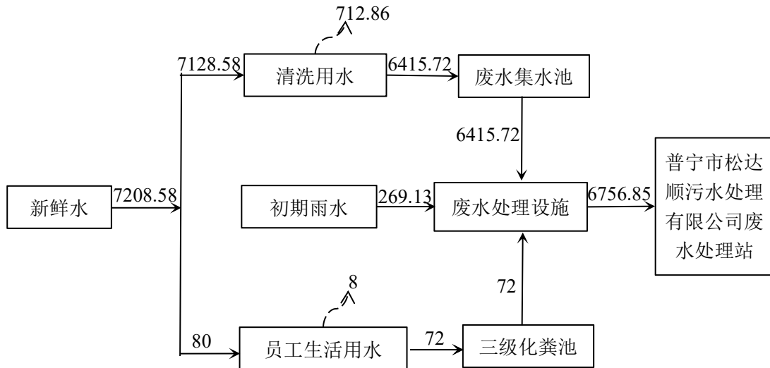
图 2-1 项目总水平衡图 (m³/a)
